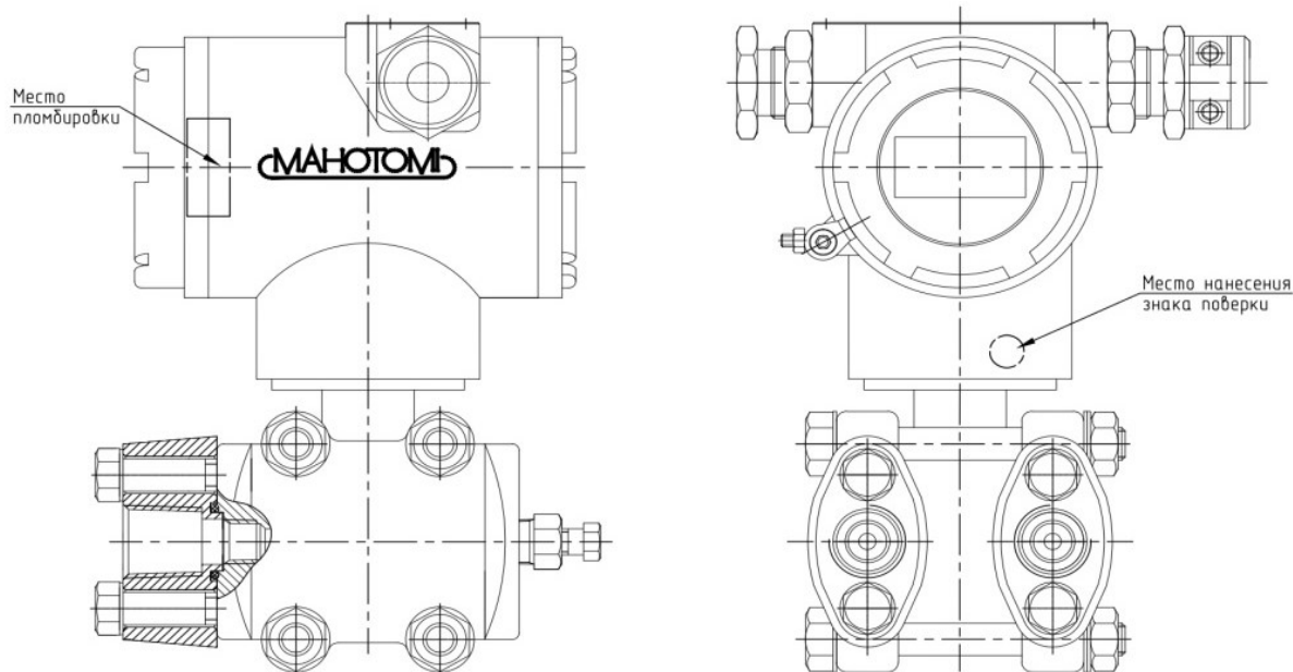
Рисунок 5 – Схема пломбировки от несанкционированного доступа внутрь и место нанесения знака поверки датчиков давления ДМ5017
